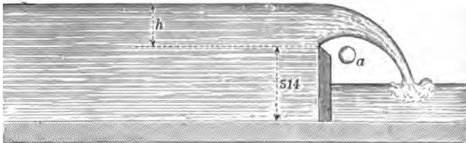
Fig. 7. Überfall ohne Seitenkontraktion.
